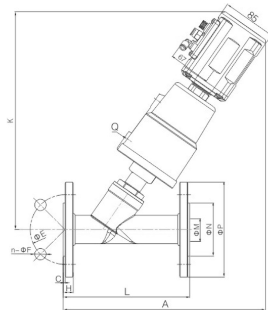
Фланцеве з'єднання
