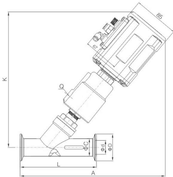
З'єднання Tri-Clamp
