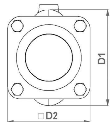
DN65 - DN100
